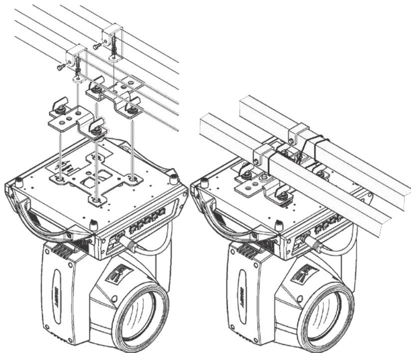
Figura 2 Instalación
