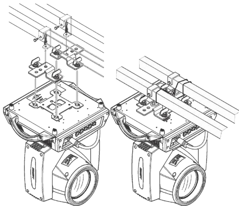
Figura 2 Instalación
