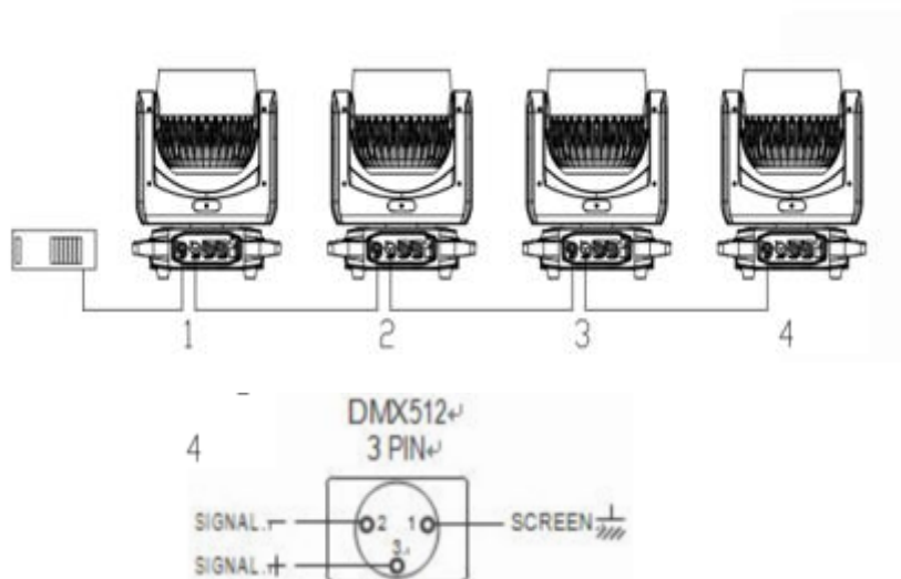
Imagen 1 Conexión de línea de señal DMX
